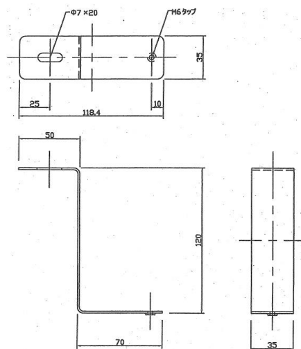
Z 金具概略図
