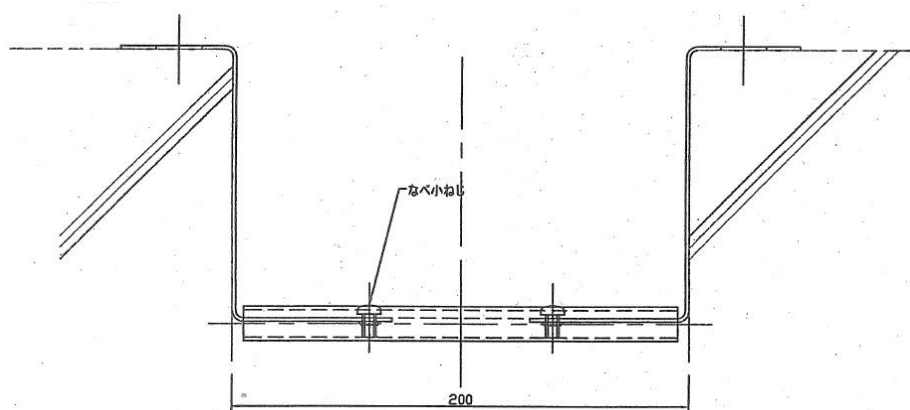
床開口内設置断面図
