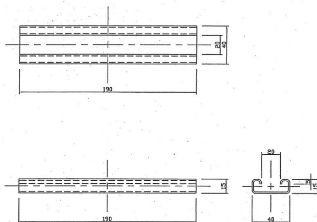
Z 金具概略図
